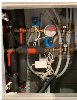
Rørskap i bad. Stoppekraner fungerer som tiltenkt
