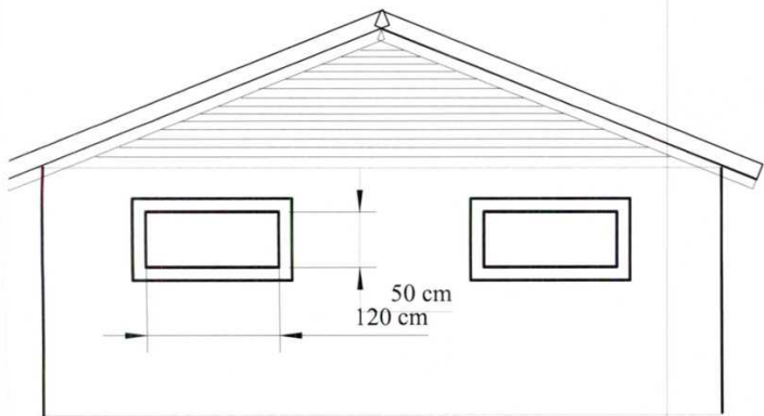
Fasade sør
