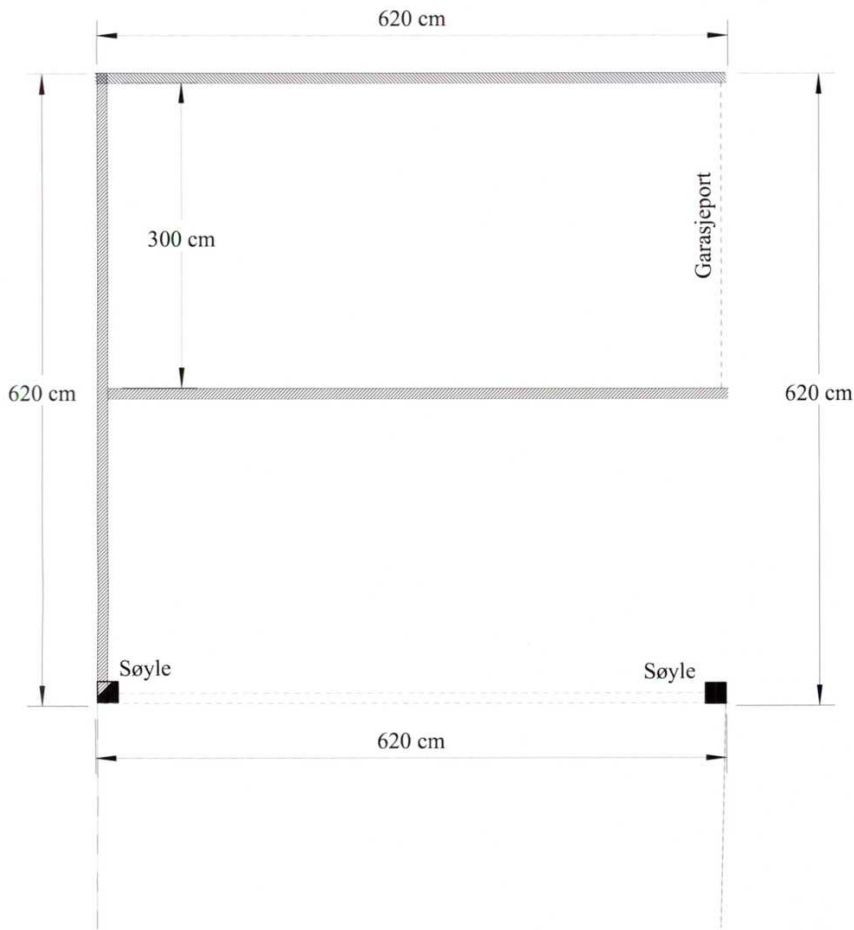
Garasje/Carport - grunnriss
