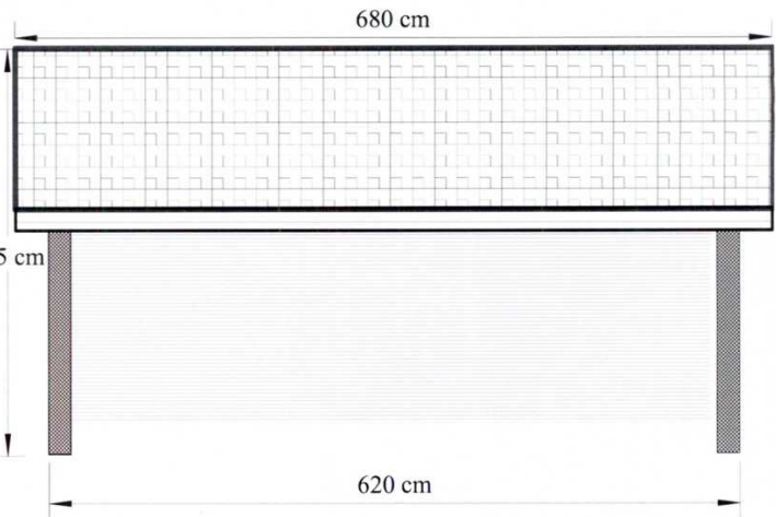
Fasade øst
