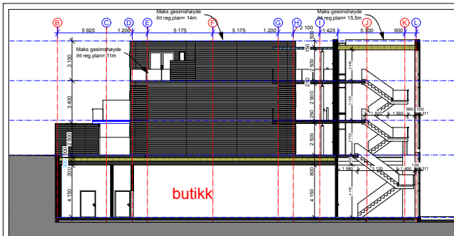
1:200 Snitt B
