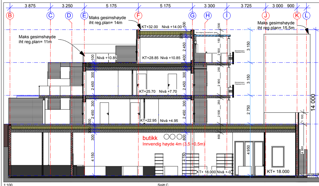
1:100 Snitt C
