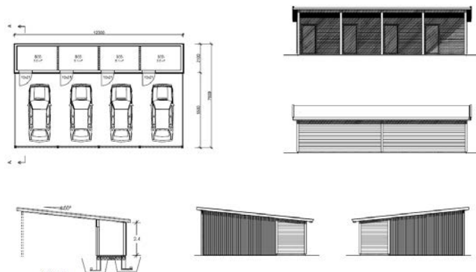
Fig. 3 Carport med bod for 4 biler – 3 stks.
