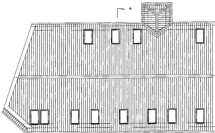
FREMTIDIG TAKPLAN
