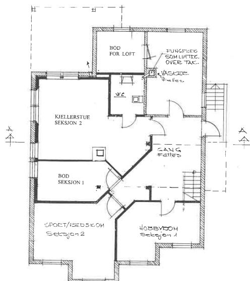
PLAN UNDERETG. (KJELLER)
