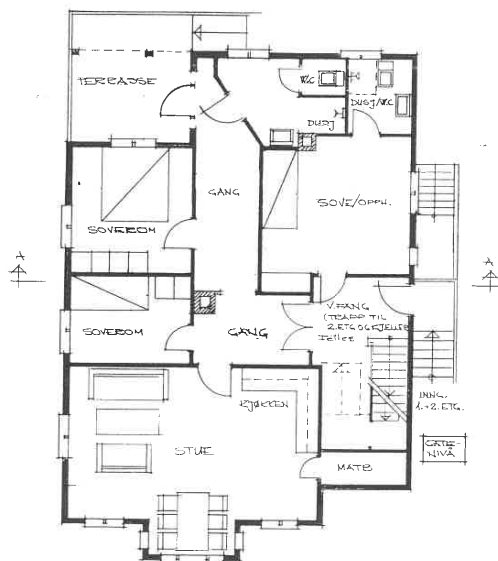
PLAN 1. ETASJE SEKJONNE 1 1/2 FELLE GANG/TRAPP
