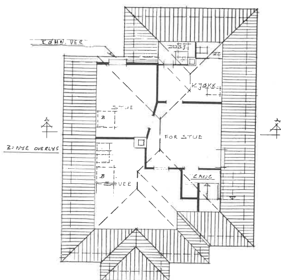
PLAN 3. ETG. LOFT SEKSJON NR. 2 (UTLEIE-ENHET)
