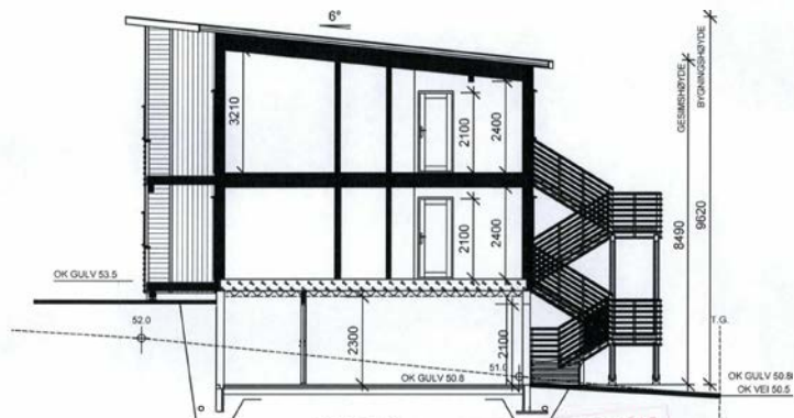
SNITT A-A
