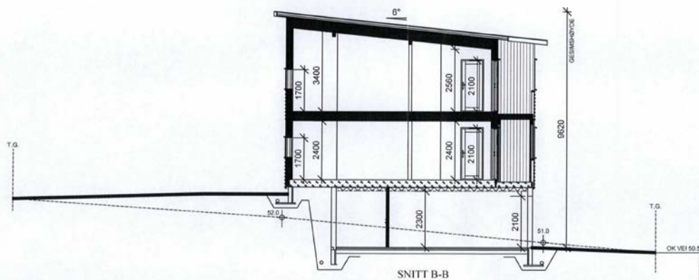
SNITT B-B
