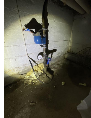
Nyere vanninntak m/varmekabel
