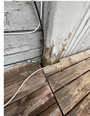
Partiell råte ytterkledning påvist
