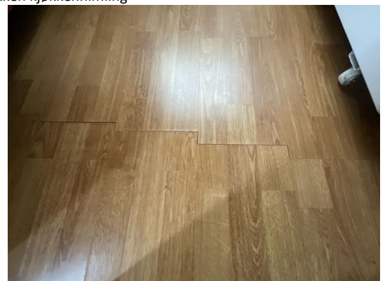
Ufagmessig laminatskjøter (ikke forskjøvet tilstrekkelig)
