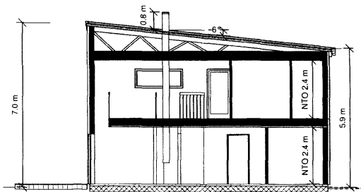
SNITT A-A
