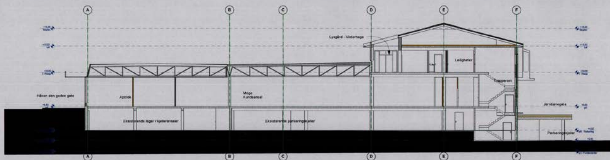
Snitt S2 - Gjennom trapperom og kundeareal
