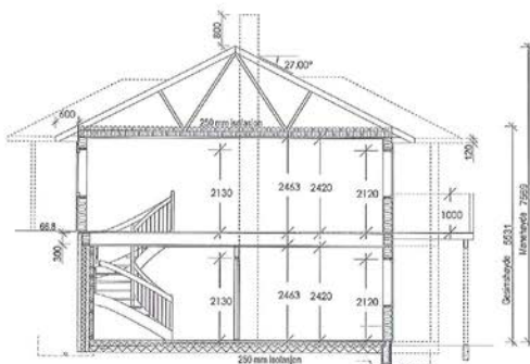
Snitt A-A
