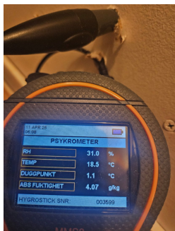
Måling av relativ luftfuktighet i veggkonstruksjon mellom bod og bad
