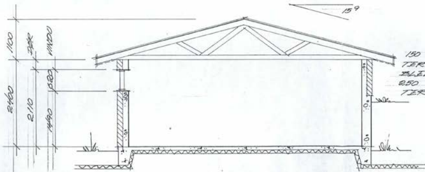
SNITT 1:50
