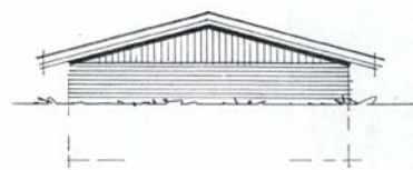
NORD 1:100
