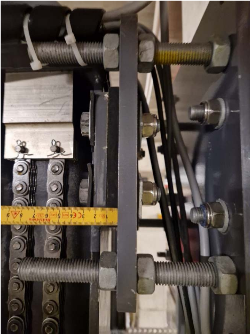
Foto 17: Demping mellom braket ca. 10 mm, og bolteforbindelse ca. 3-4mm
