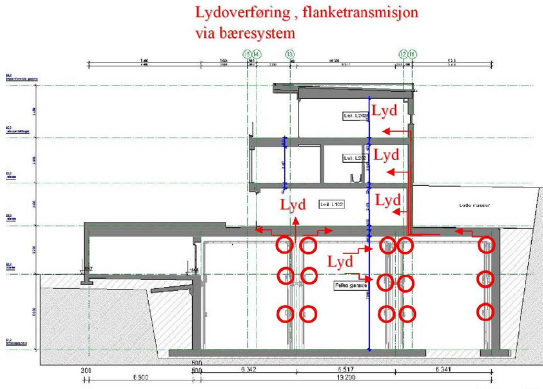
Figur 12: Prinsipp for flanketransmisjon av lyd i parkeringsanlegg BK2 (Hus L), snitt C. Dette er et utsnitt fra figur 3 (Tegning I_a29_02_snitt_og_fasader_pdf, lastet ned fra Asker kommune)
