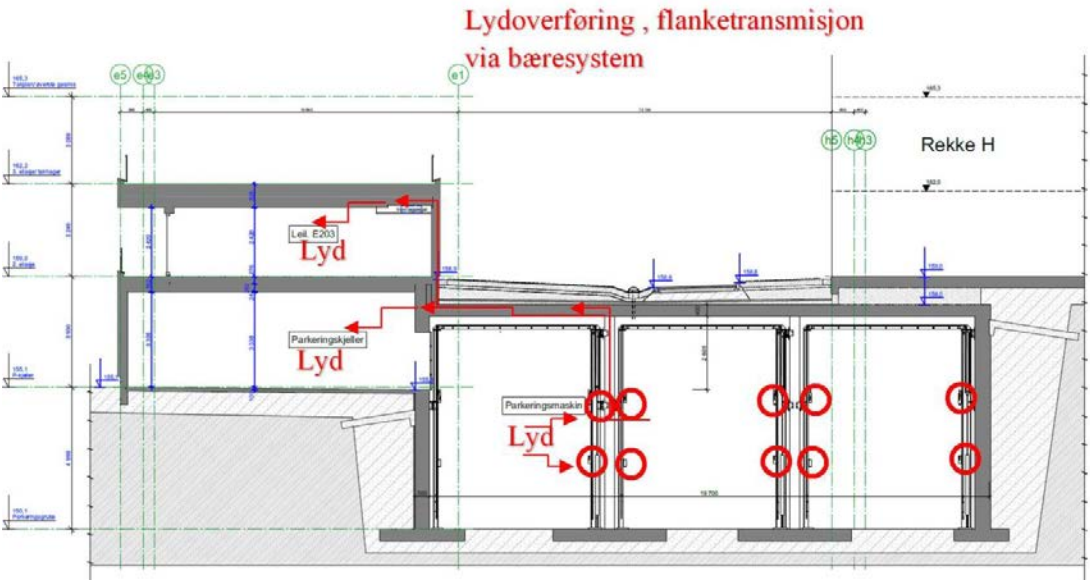
Figur 11: Prinsipp for flanketransmisjon av lyd, parkeringsanlegg BK1 (Hus E). Dette er et utsnitt fra figur 1 (e_a29_02_snitt_og_fasader_pdf, lastet ned fra Asker kommune).
