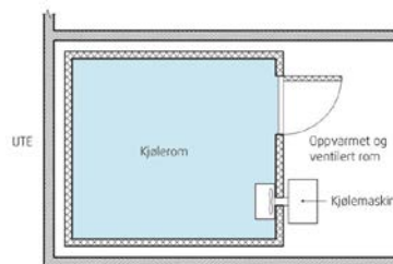
Fig. 71 Plan-skisse av et mindre, innbygd kjølerom av prefabrikkerte kjøleroms-elementer
