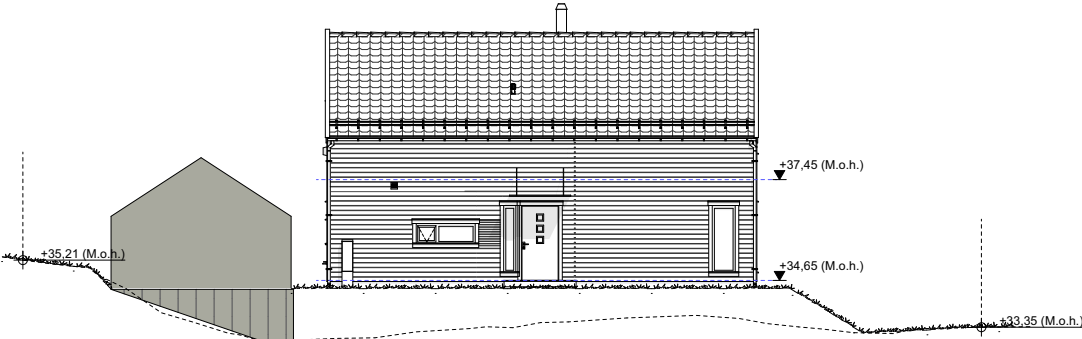
(1) Fasade Øst
