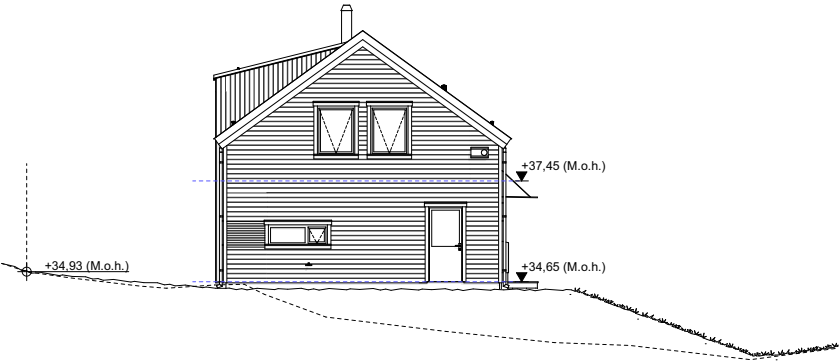
(2) Fasade Sør
