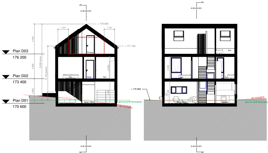
Snitt D1 1 : 100
