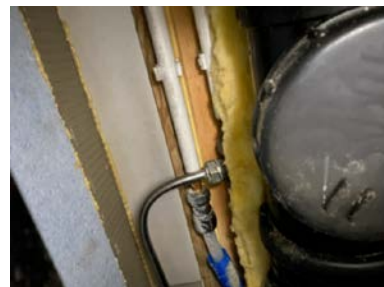
Det er ikke montert tettemuffer i enden av varerør i rørsjakt på badet.
