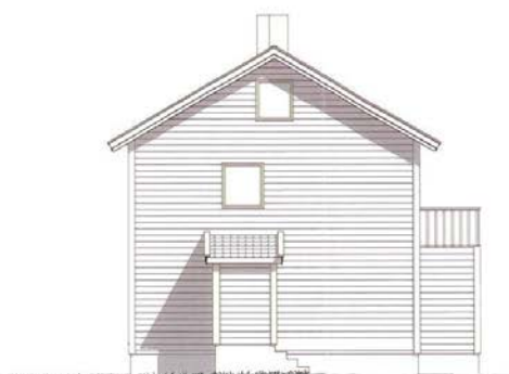
FASADE NORD
