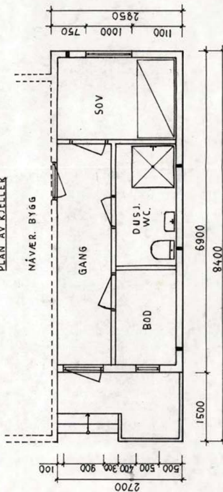
PLAN AV 1. ETASJE
