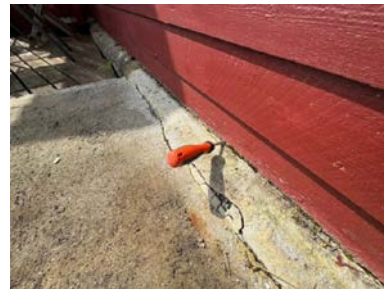
Eksempel på råteskadet kledning og ingen ventilering av kledningen.
