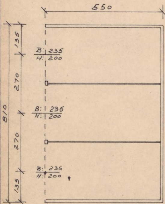
Grunnplan-garasje.
