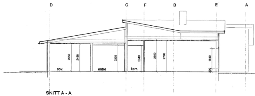
SNITT A - A
