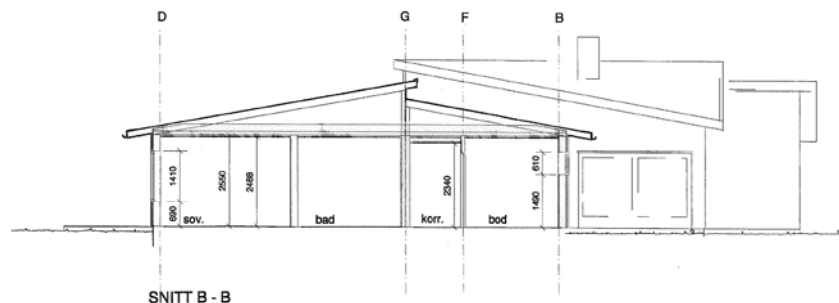
SNITT B - B
