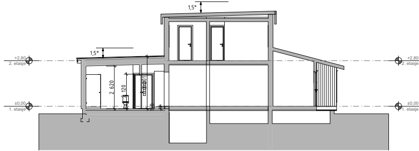
A1 Snitt
