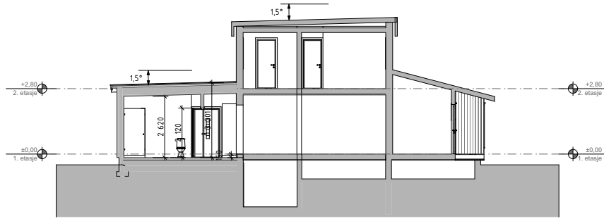
A1 Snitt
