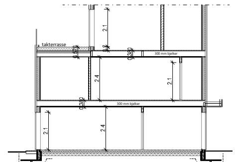
Snitt E-E
