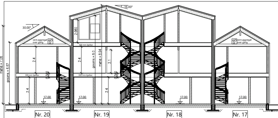
Snitt A-A
