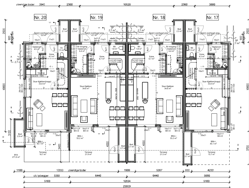
Plan 1. Etasje
