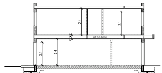
Snitt C-C
