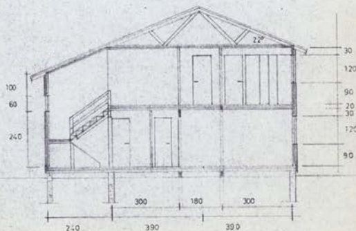
SNITT A-A
