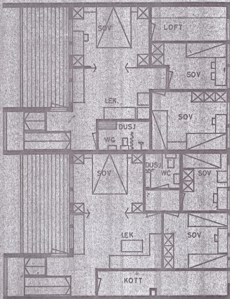
PLAN 2. ETG.
