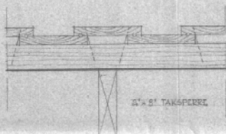
DETALJ 1. M=1:5
