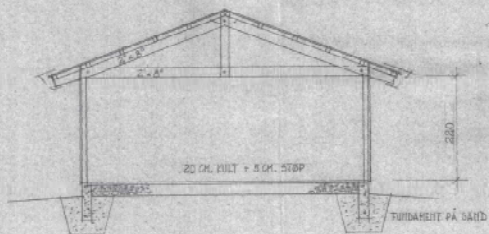
SNITT
